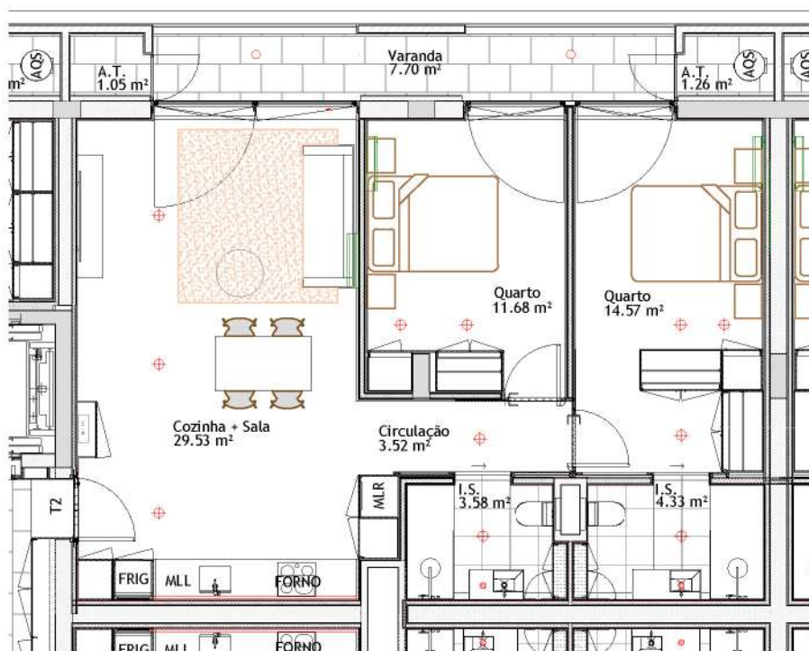
Planta da Fração
